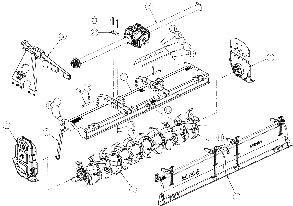
AR6280H
